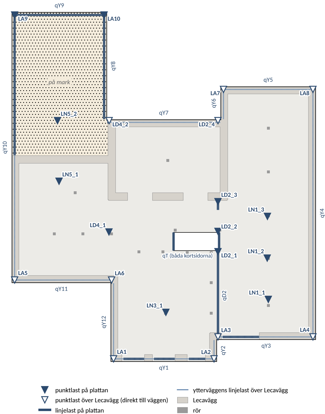
Figur 2: Laster från plan 1. Punktlasterna heter efter balken de kommer från (LN1_1 = nockbalk 1, första stolpen räknat från balkens början vid lägst y), LA1–LA10 är hörnstolpar. Linjelaster: ytterväggar qY1–qY12, dalbalk 2 via vägg qD2, trappan qT.
