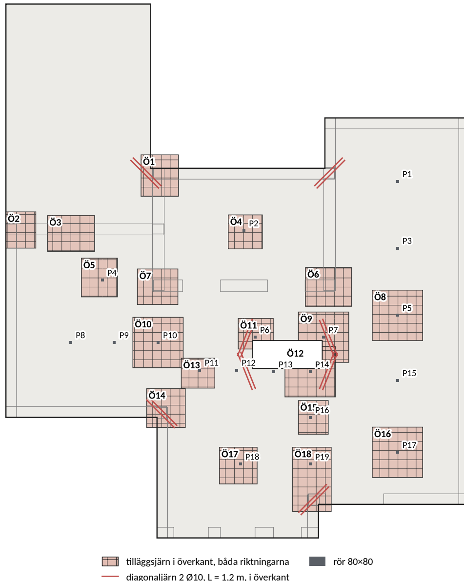
Figur 4: Tilläggsjärn i överkant och diagonaljärn. Zonerna omfattar området där nätet inte räcker plus 0,4 m förankring, och 1,5 × 1,5 m kring rör som behöver mer armering för genomstansning eller där tillägg föreskrivs (P7, P14, P17).
